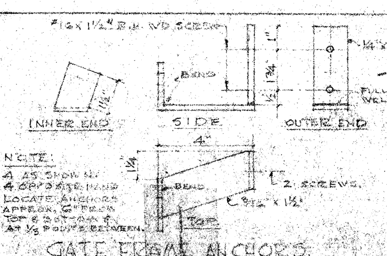
GATE FRAME ANCHORS SCALE: 1/4" = 1'-0"
